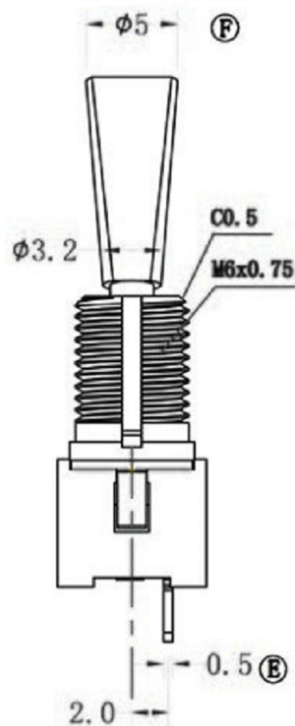
标注 A - F 为重点尺寸
